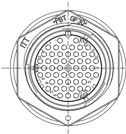
插入面视图
