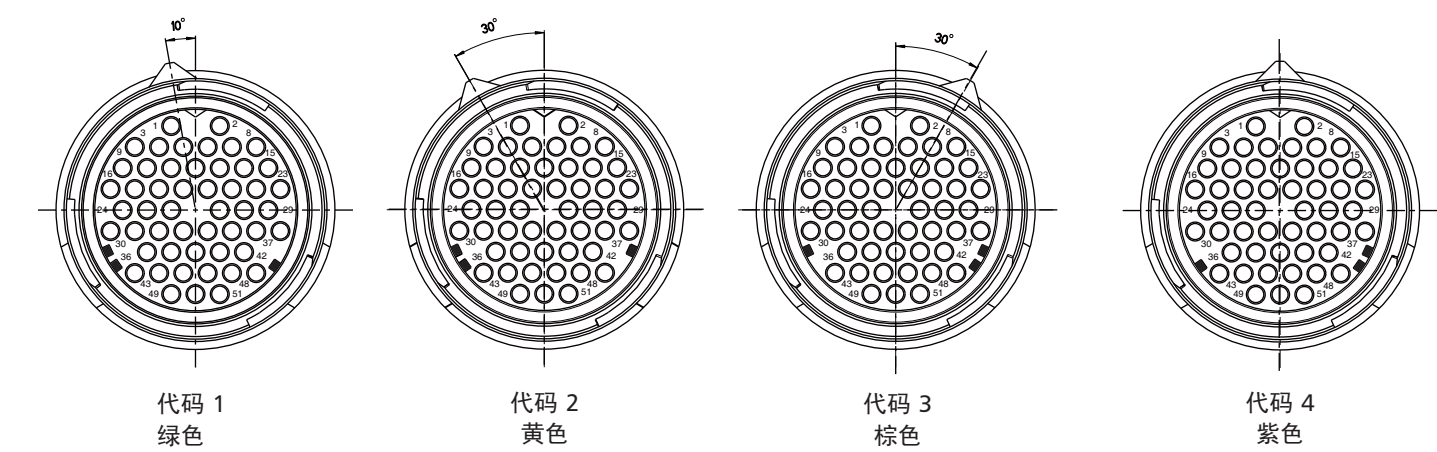
插合面视图
