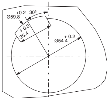
墙面厚度 标准锁紧螺母：最小 1,5/最大 4,0mm
