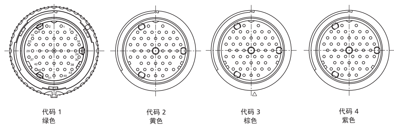
插合面视图
