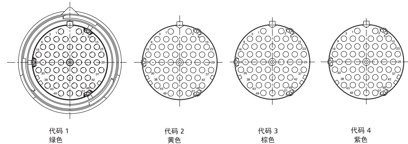
插合面视图
